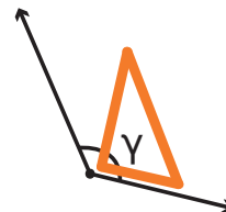
αμβλεία γωνία
